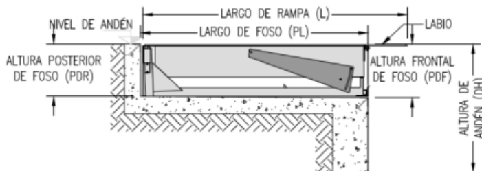
Vista Lateral
