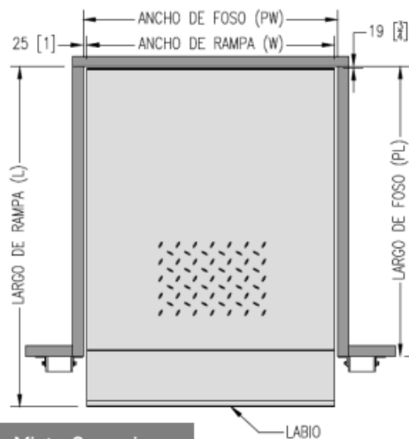
Vista Superior
