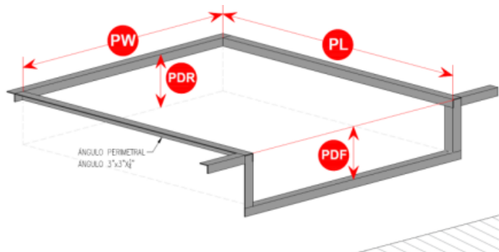
Isométrico Foso
