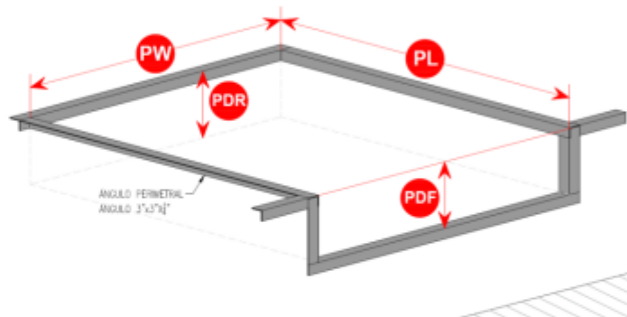
Isométrico Foso
